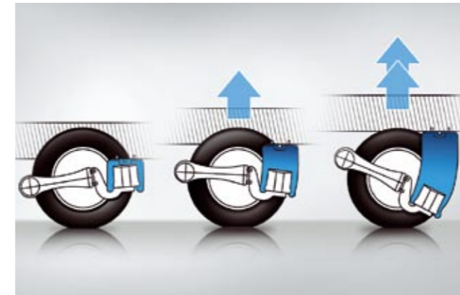
Düşük araç yüksekliğinin yanı sıra büyük kalkma aralığı Large lift range with a low ride height
