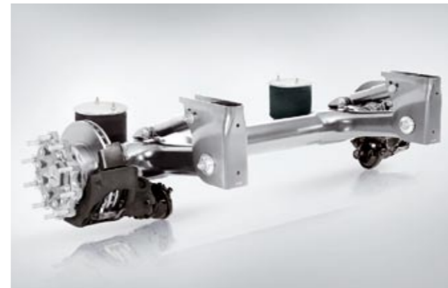
Güzel form verilmiş tasarımda hafif, sağlam ve güvenilir Lightweight, robust and reliable with an elegant design
