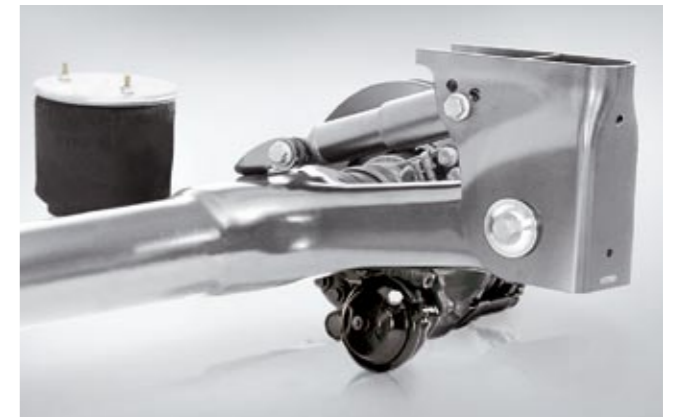
Aks gövdesine entegre edilmiş boyuna buğu kolu, aks kovanı fren flanşı ve aks başı
